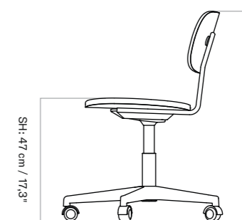
H: 78,5 cm / 30,9"
